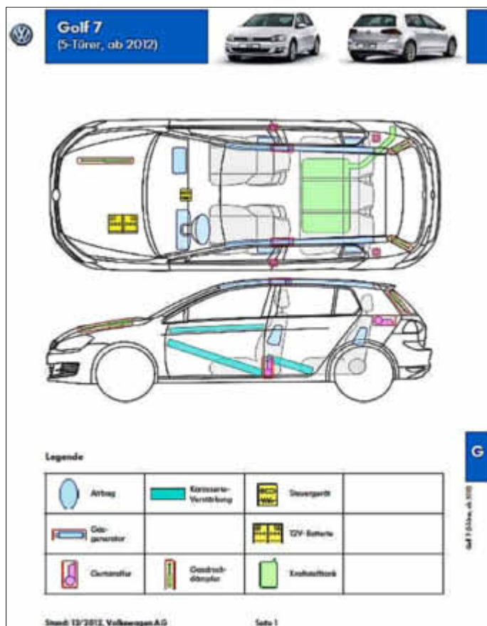
Rettungskarte VW Golf
