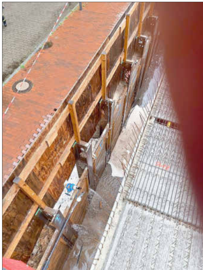
Blick von der Drehleiter auf den Wassereinbruch, der den Gehweg abrutschen ließ.
