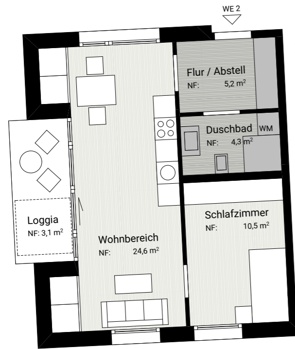
Wohnheit 2, Erdgeschoss Zwei-Zimmer-Wohnung, barrierefrei, 48 m 2
