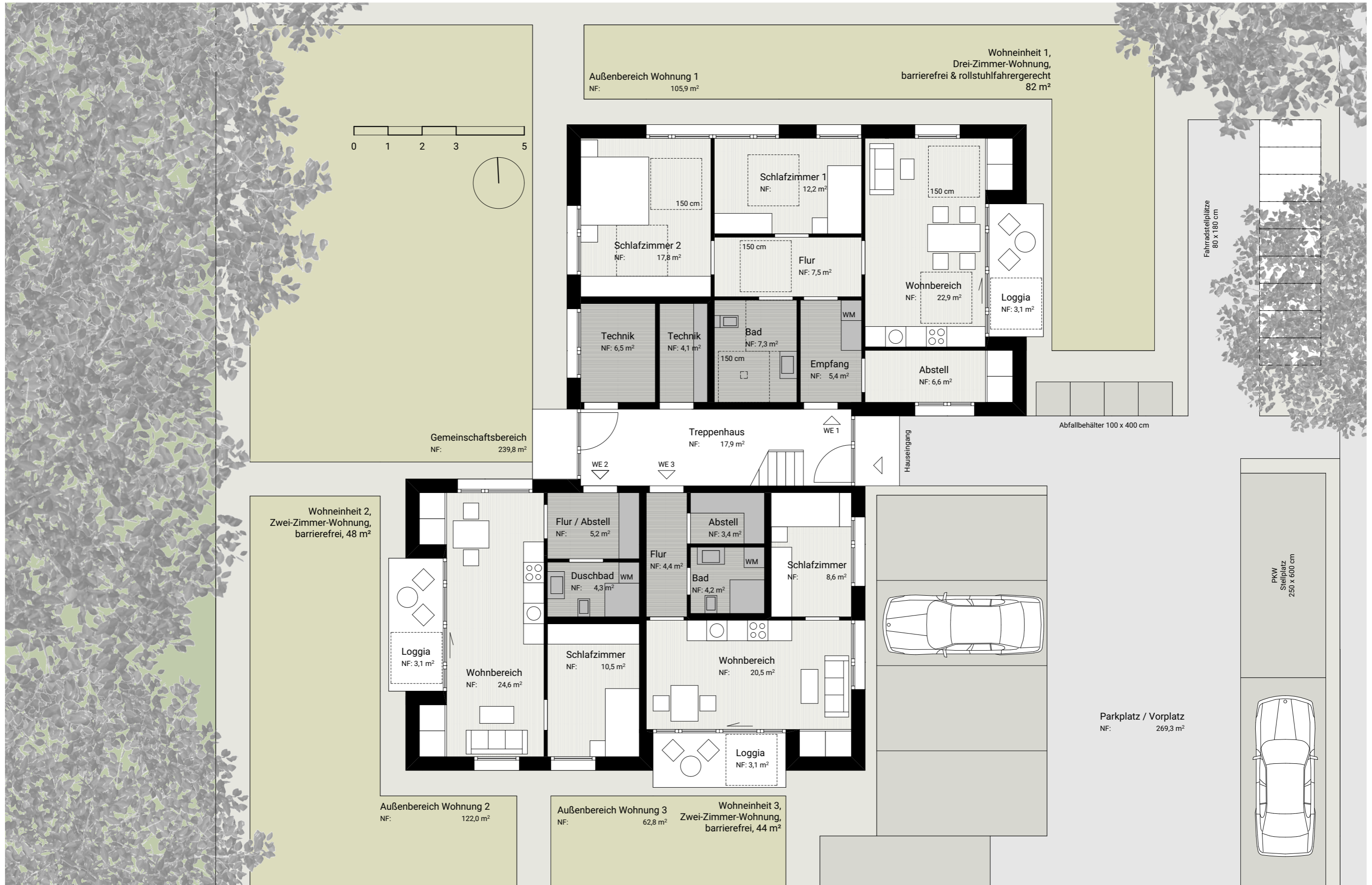
Grundriss Erdgeschoss 1:100
