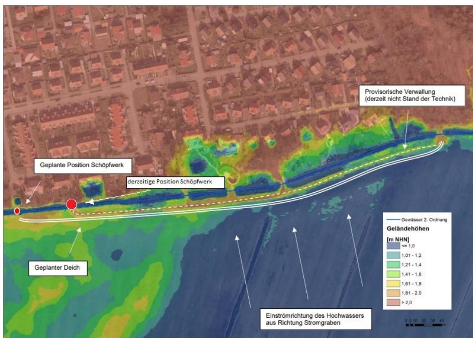
Abbildung 2-2: Vermessungsergebnisse 02/2021 und Geländemodell im Bereich Tabakwiese/Graal-Müritz und nördlich angrenzende Bebauung Koppenheide
